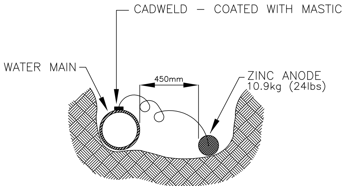
ZINC ANODE
