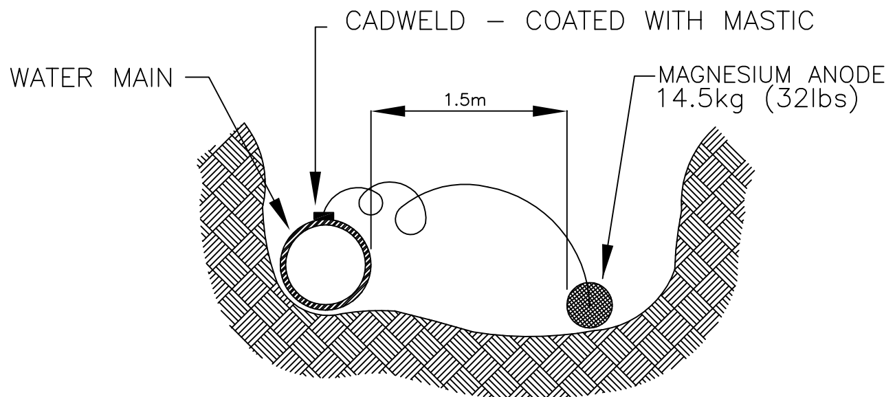
MAGNESIUM ANODE
